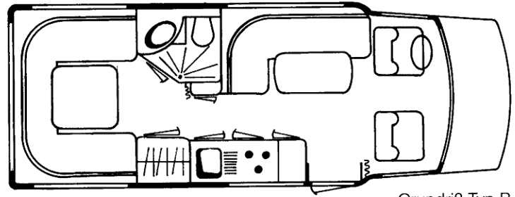
Grundriß Typ B
