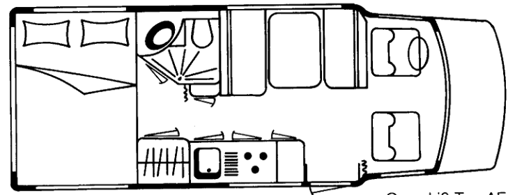
Grundriß Typ AF
